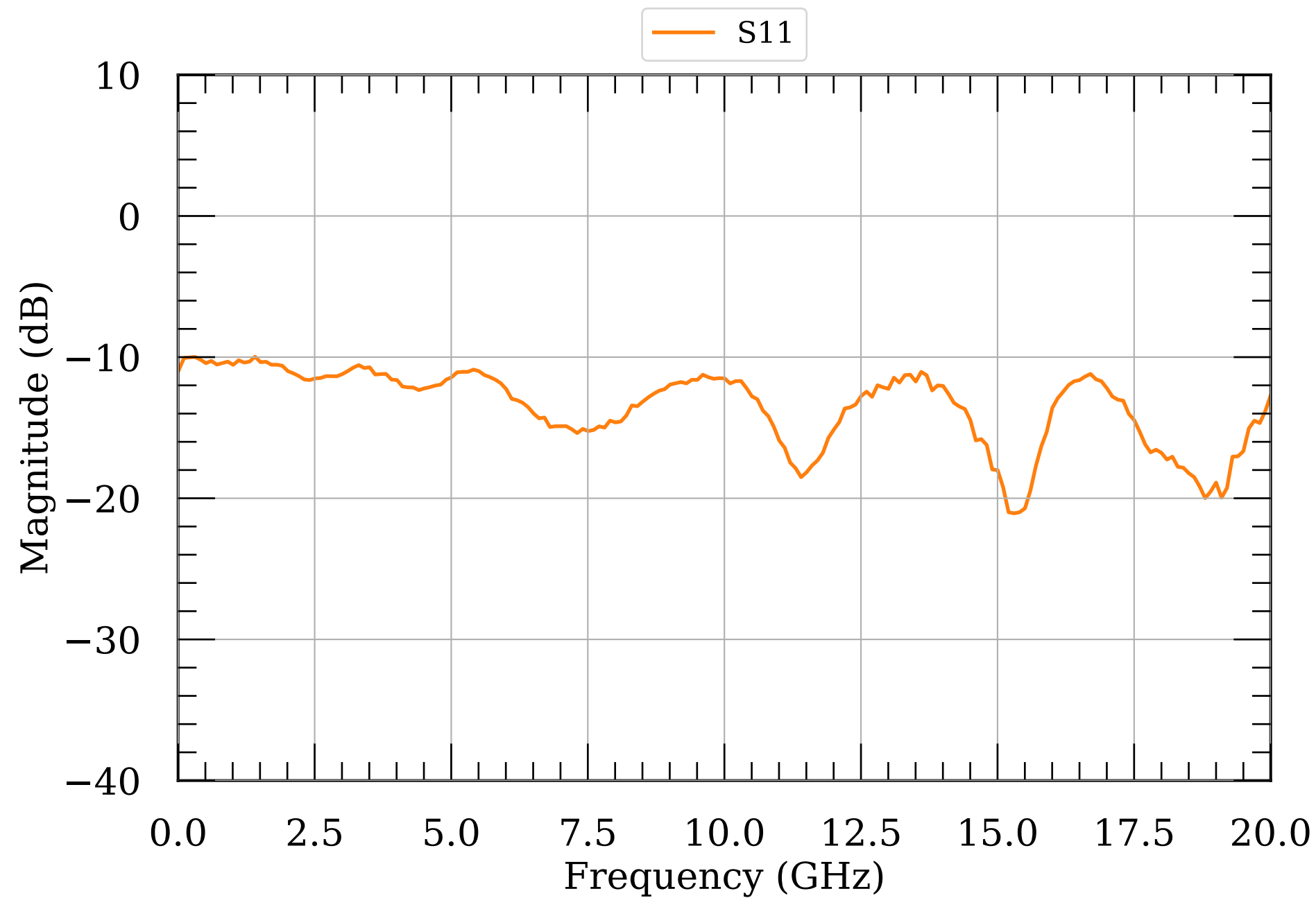
LNA S-params module093
